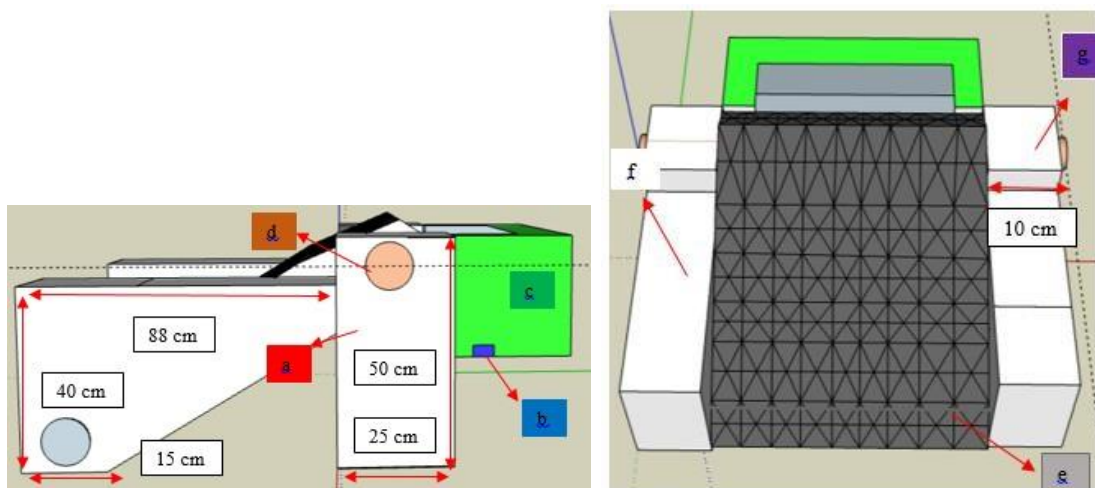
Gambar 3. Desain Alat
