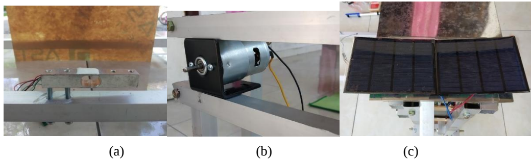
Gambar 5 Pemasangan Sensor Load Cell (a), Pemasangan Motor DC (b), dan Panel Solar sel (c)
