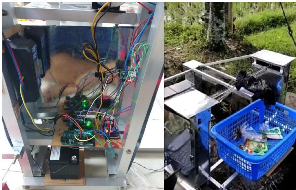
Gambar 6 Pemasangan Arduino, Modul GSM, Modul Step Down Buck Conveter, Driver Motor L298N, Mikrocas dan Baterai Aki.
